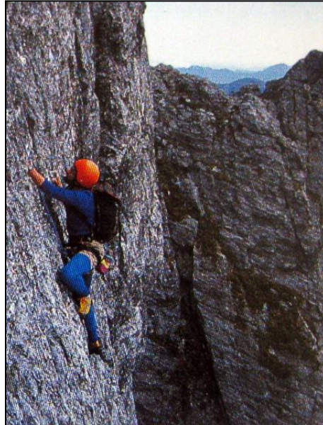
Dolerita.
