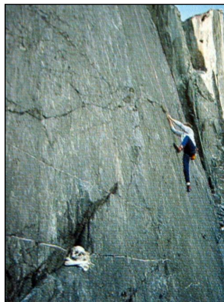
Pizarra.
