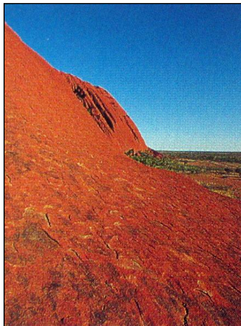
Cuarcita.
