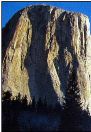
Granito
